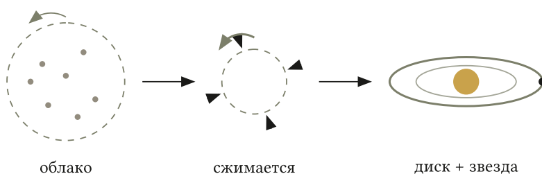
Рис. 1. Вращающееся газопылевое облако под собственным тяготением сжимается, раскручивается и сплющивается в диск; в центре загорается звезда, из диска собираются планеты.
