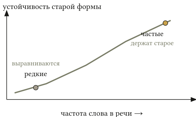
Рис. 1. Чем чаще слово встречается в речи, тем дольше оно сохраняет старую неправильную форму; редкие слова быстрее переходят на общее правило.
